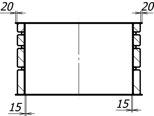
F-F (1 : 30)
